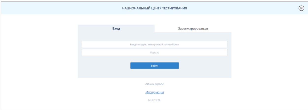
Рисунок 2 - Страница авторизации/регистрации
